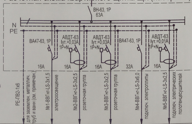
Расчетная схема квартирного щитка ШК (наборный)
