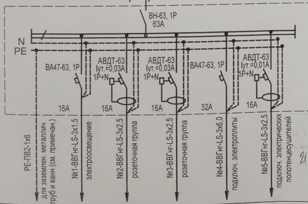
Расчетная схема квартирного щитка ЩК (наборный)
